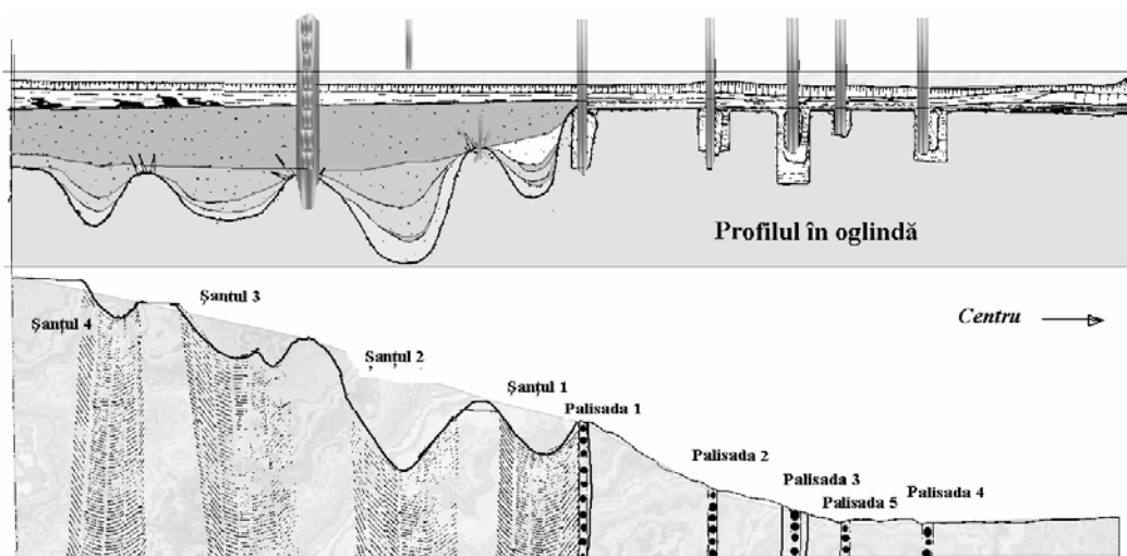
Fig. IIIb.199. Parja, sistemul de fortificații din marginea de N a stațiunii; jos planul, sus profilul
