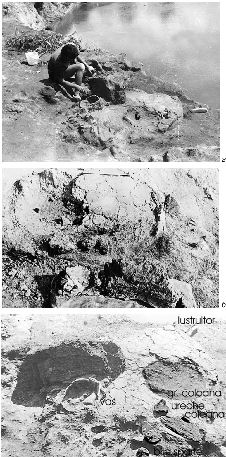
Fig. IIIb.185. Parja, P126, caseta cu vas spart în spate, cuptorul cu gaura de coloană
