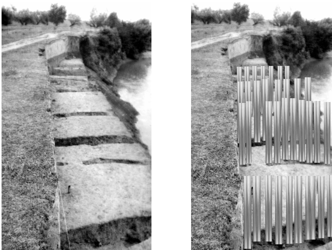
Fig. IIIb.206. Parja, palisadele: a) ▲ vedere spre nord; b) reconstruire ▲
