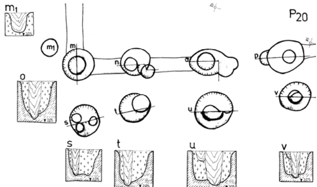
Fig. IIIb.170. Parja, Casa Tribului, structuri de fundații: a) partea de E; b) gropi de stâlp
