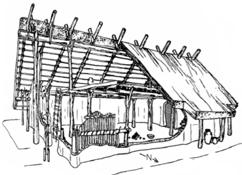
Fig. IIIb.174. Parja, barjă sau „Casa Tribului”, P20, reconstituire
