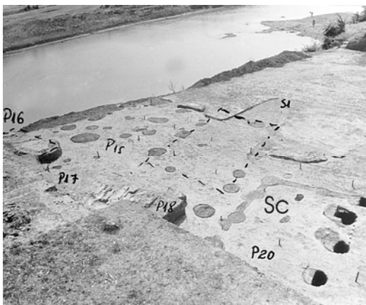
Fig. IIIb.170. Parja, Casa Tribului, structuri de fundații: a) partea de E; b) gropi de stâlp
